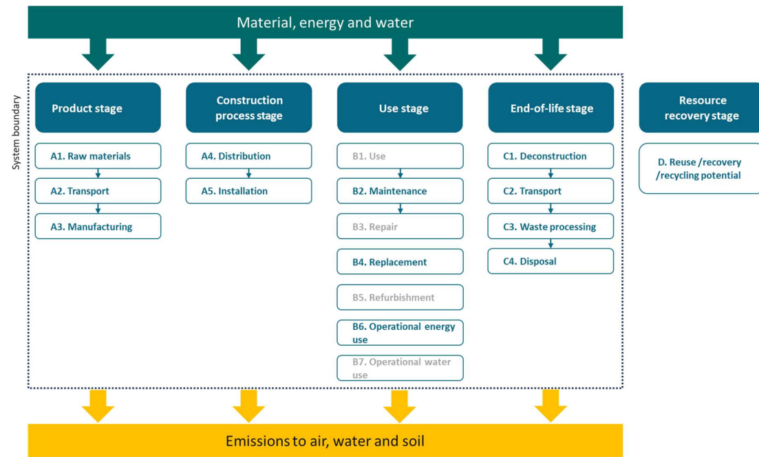
SECTO 4200 SYSTEM DIAGRAM
