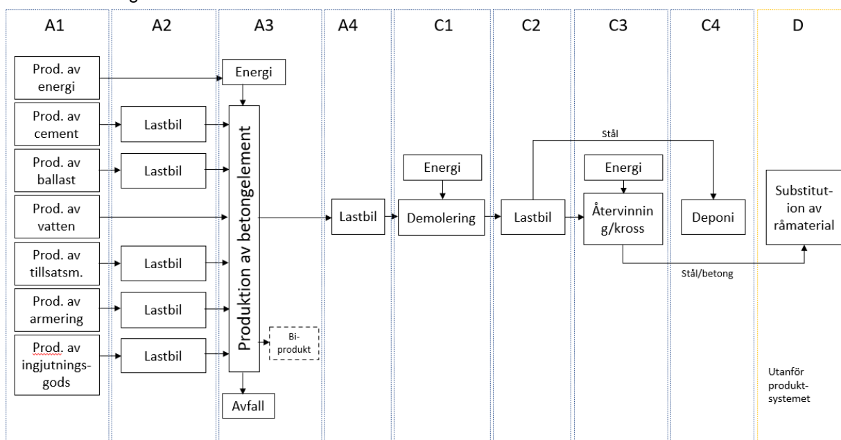
Figur 2 Flödesschema
