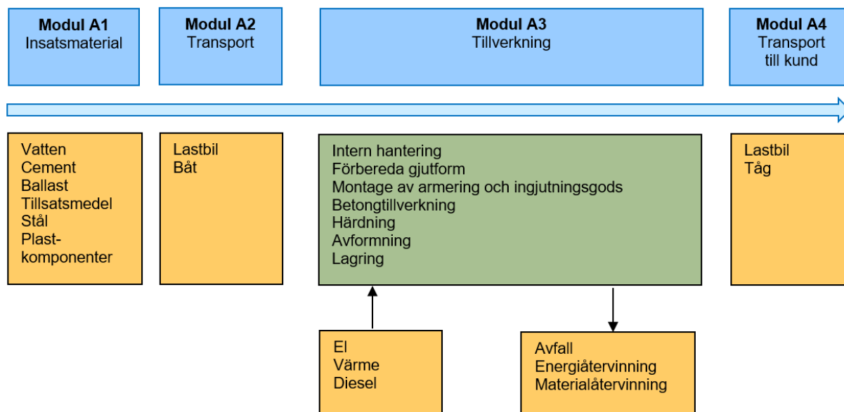
Figur 2 Flödesschema
