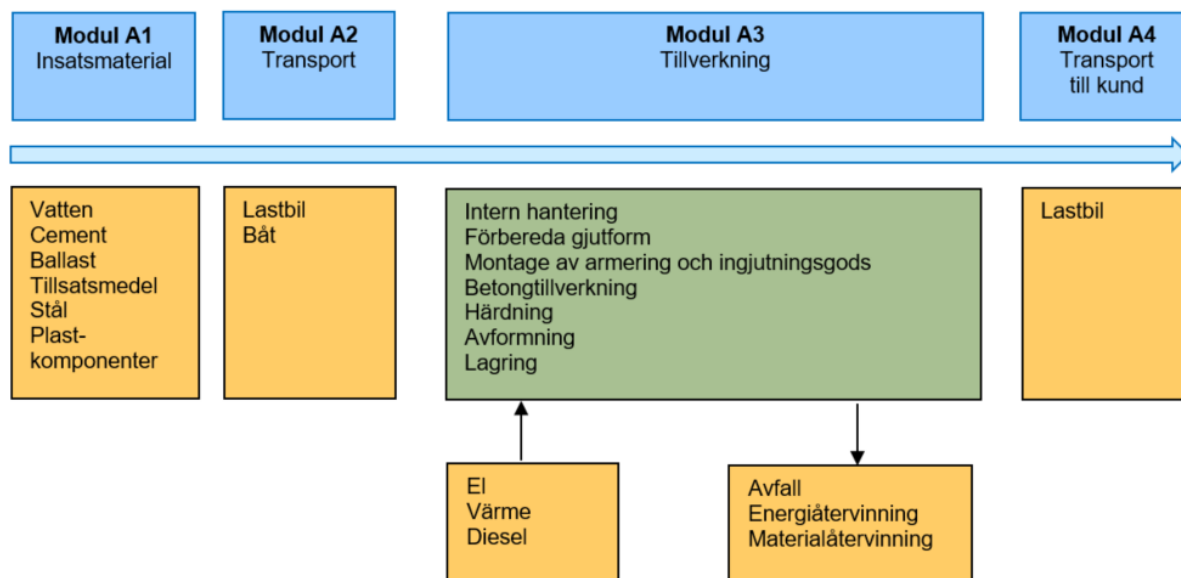
Figur 2 Flödesschema
