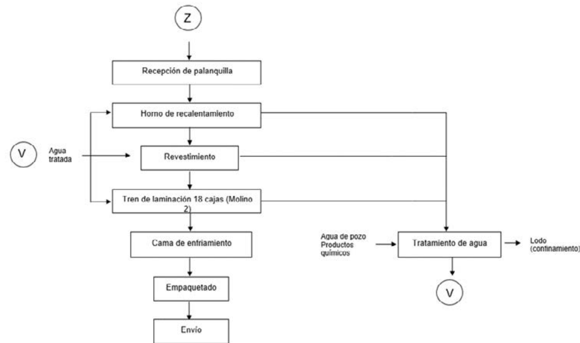
Figura 3. Diagrama de flujo del tren de laminación para la fabricación de varilla a partir de chatarra por parte de T A 2000.
